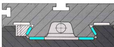
2 Guide a coda di rondine
