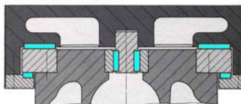
2 Guide a coda di rondine
